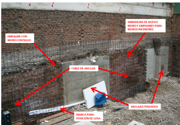
Figura 3. Paneles secundarios en proceso constructivo del muro anclado. Foto obra “Edificio Cipreses”.
