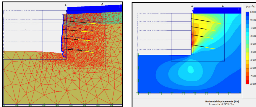
Figura 7. Izq.: Deformación del modelo de EF después del cálculo en PLAXIS (ampliada 200 veces). Der.: Rango de deformaciones obtenidas en el modelo de EF.
