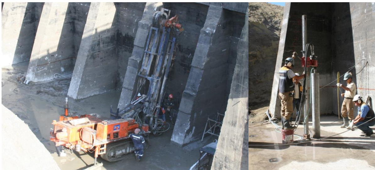
FIGURA 3 Ejecución de perforaciones con diamantina y de micropilotes autoperforantes.
