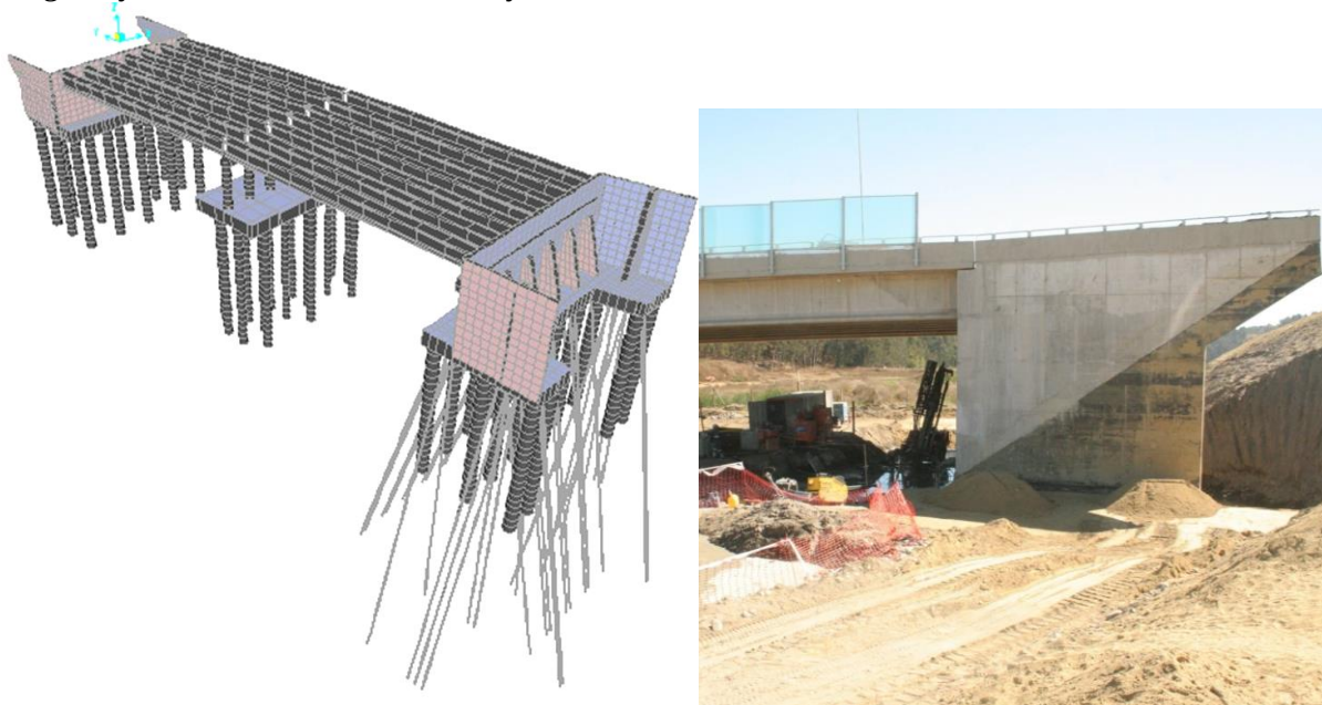
FIGURA 2 Refuerzo del estribo con micropilotes Ischebeck Titan 103/78.
