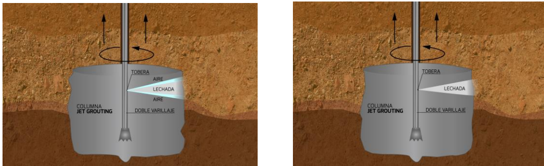
FIGURA 9 Ejemplos de sistemas de Jet I (monofluído) y jet II (doble fluido).
