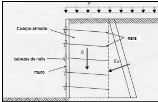
Figura 11. Idealización del cuerpo de tierra armado con soil nailing
