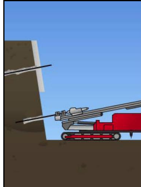
Figura 8. Esquema de ejecución del Soil Nailing
