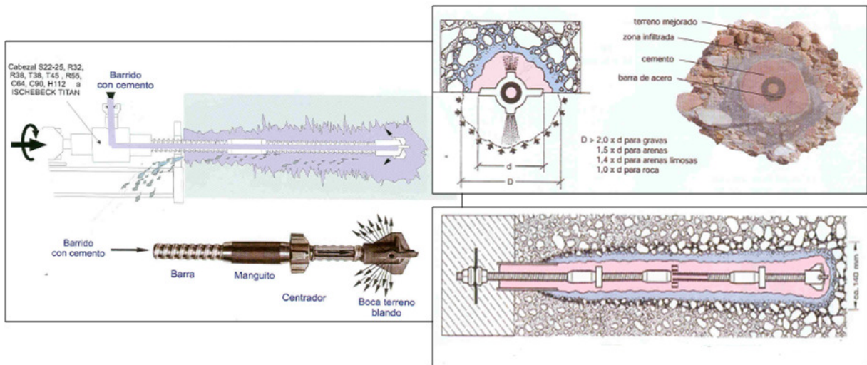
Figura 6. Detalle constructivo de los anclajes pasivos del tipo TITAN autopercutores
