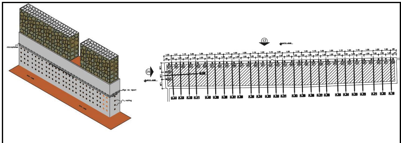
Figura 10. Esquema de distribución de nails y micropilotes
