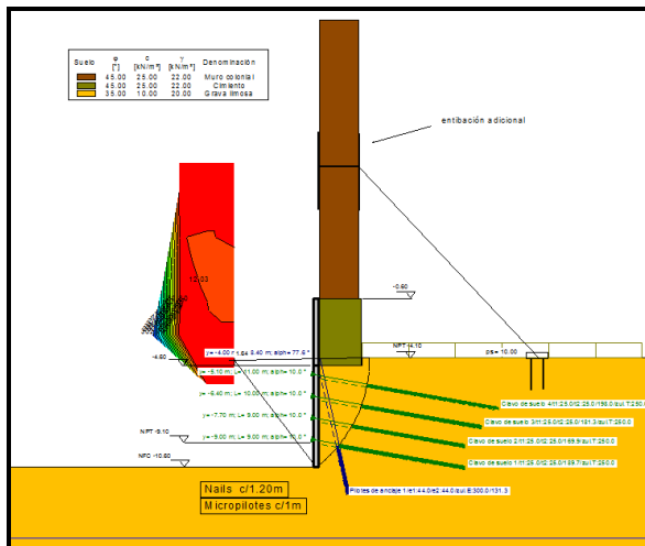
Figura 12. Verificaciones de estabilidad mediante el programa GGU-STABILITY
