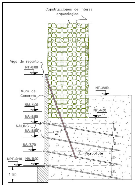
Figura 7. Esquema de los elementos de sostenimiento
