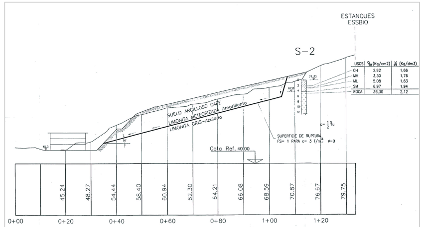
Figura 3 - Perfil de la falla. Se aprecia las unidades de suelo presentes y el contacto Limonita (arenisca) – Arcilla, donde se produjo el deslizamientos.
