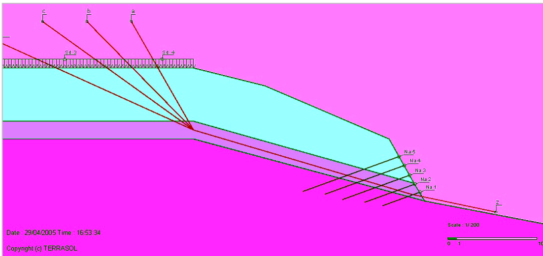
Figura 6 - Modelo de cálculo empleado para el diseño.
