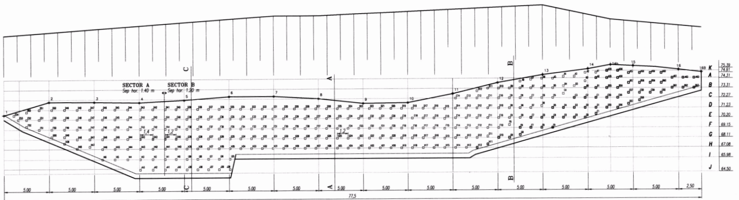
Figura 7 - Elevación y corte de la solución adoptada.
